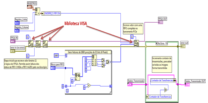
Figura 13: Programa desenvolvido em linguagem gráfica
