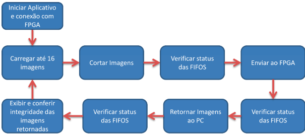
Figura 17: Esquema para teste de transferência das imagens
